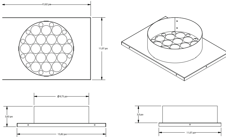
Fig. 1 – Détail dimensionnel de la transition de l'ouverture carrée à ronde
